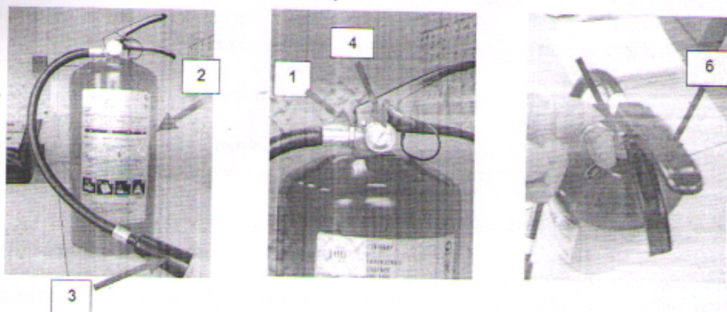
Рис.1. Порошковый огнетушитель типа ОП-4(3)
